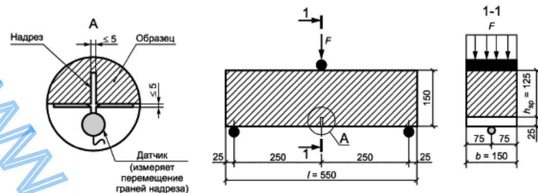
а - При измерении перемещения внешних граней надреза
